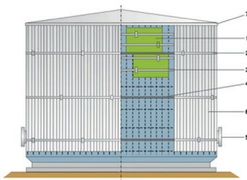
Figura 4.7.1. Ejemplo de aislamiento en tanque de almacenamiento
