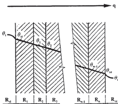
Figura C.16. Distribución de temperatura en una pared plana multicapa, mostrando la dependencia lineal de la resistencia térmica superficial y las resistencias térmicas de cada capa independiente.
