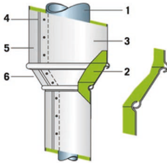
Figura 4.9.3.A. Ejemplo de reducción vertical (1: Tubería vertical - 2: Aislante - 3: Revestimiento metálico exterior - 4: Tornillo autoroscante o remache. 5: Junta - 6: Reducción).
