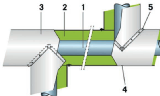
Figura 4.9.2.D. Ejemplo de insertos (1: Tubería - 2: Aislamiento - 3: Revestimiento metálico exterior - 4: Orificio para drenaje - 5: Sellado de junta con masilla impermeable).
